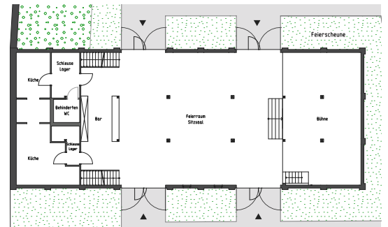
Grundriss Erdgeschoss
